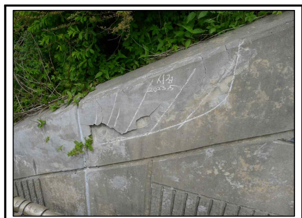
사진번호 72 갱구부 옹벽(시점 좌측) 보수부 들뜸, 박락 외관망도 16-1
