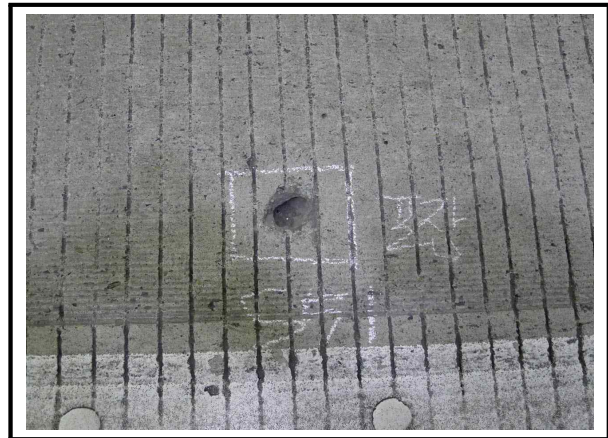
사진번호 68 포장부 S51 패임 외관망도 11-18
