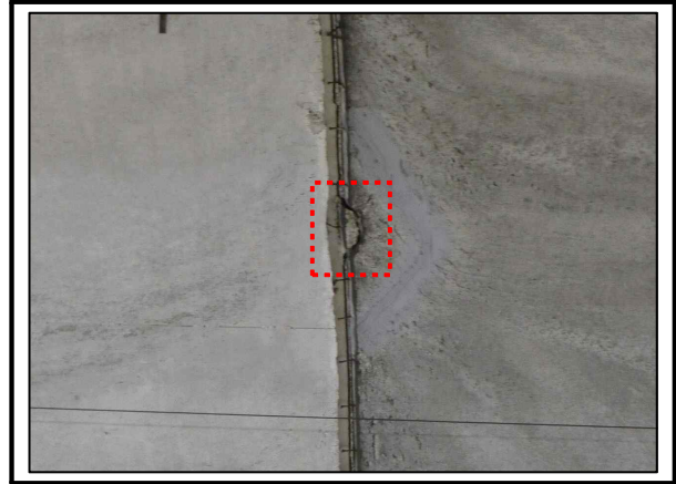
사진번호 26 천단부 S50(J50) 외관망도 10-22 시공이음부 박락
