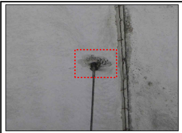
사진번호 27 천단부 S56 외관망도 12-22 파손(조명시설 앵커 주변)
