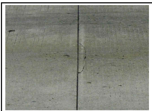
사진번호 65 포장부 S24 줄눈 주변 파손 외관망도 5-19
