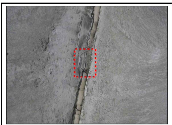
사진번호 23 천단부 S44(J44) 외관망도 9-17 시공이음 보수부 박락
