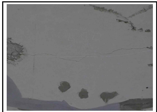
사진번호 30 천단부 S70 외관망도 14-1 균열(0.3mm 미만)
