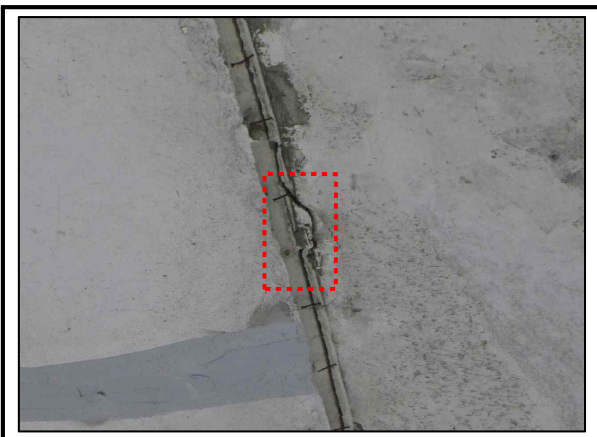
사진번호 29 천단부 S67(J67) 외관망도 14-16 시공이음부 박락
